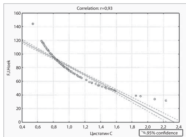
Рис. 2. Кореляційна залежність рШКФц від рівня ЦсС за рівнянням F.J. Ноєк і співавт.
