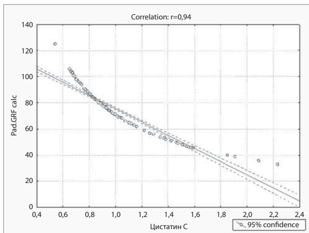
Рис. 3. Кореляційна залежність рШКФц від рівня ЦсС за рівнянням Pediatric GFR Calculator — NKF
